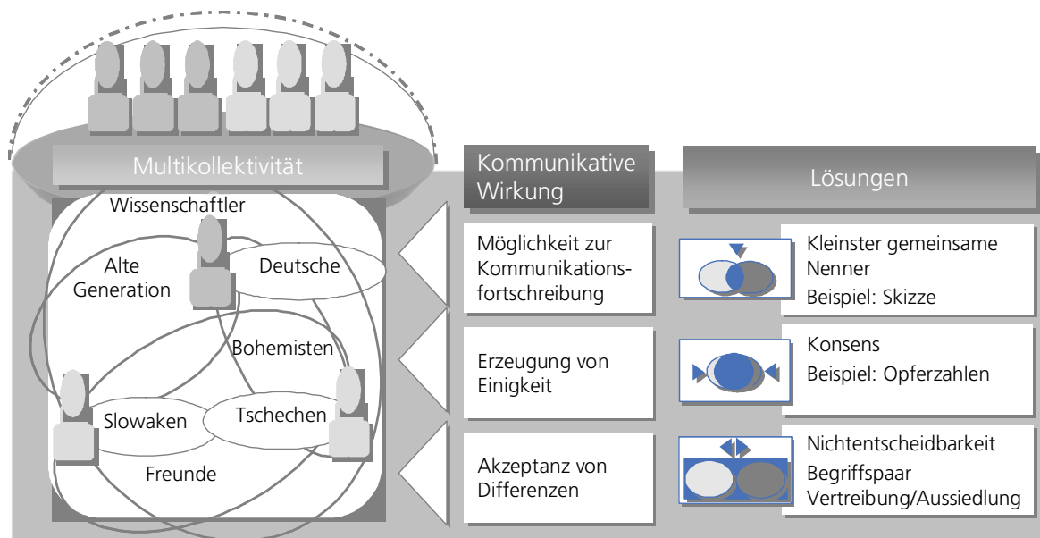
Abb. 3: Iterative Stabilität
